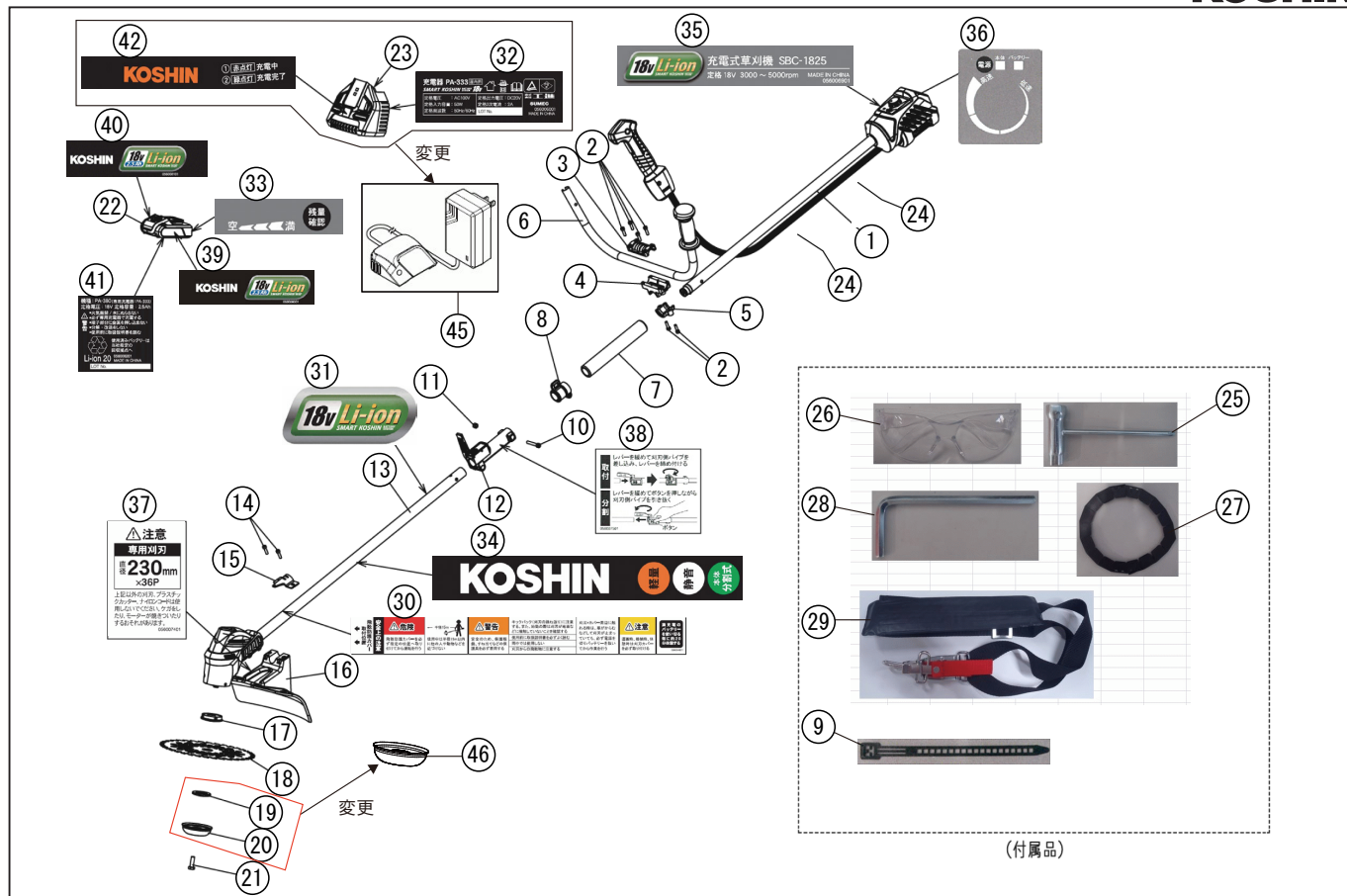
型式名 SBC-1825-AAA-3 (056851206)
