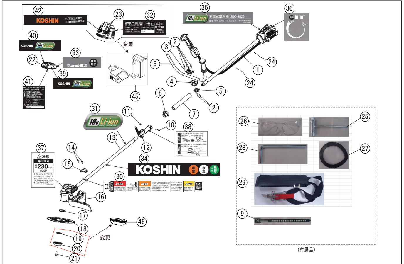
型式名 SBC-1825-AAA-3 (056851206)
